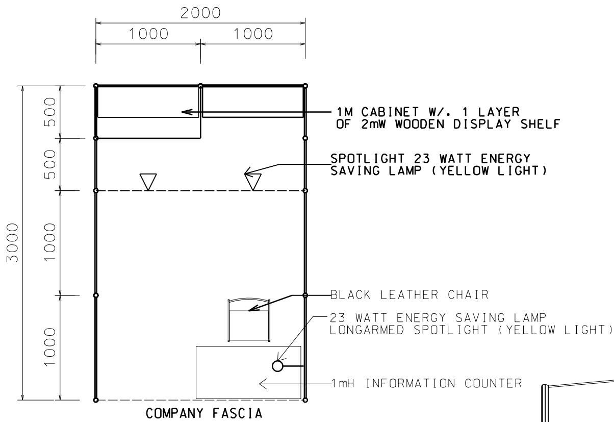
PLAN 2M(W) X 3M(D) X 2.5M(H)
