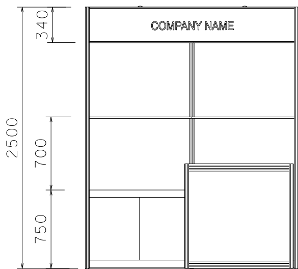
ELEVATION 2M(W) X 3M(D) X 2.5M(H)
